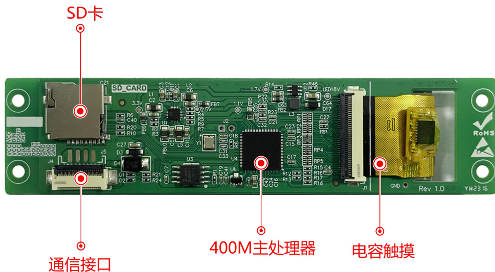
图 1-3 硬件配置图
