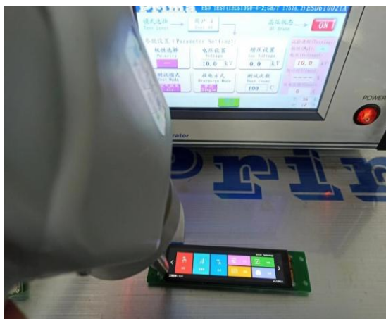
图 3-2ESD 测试图
