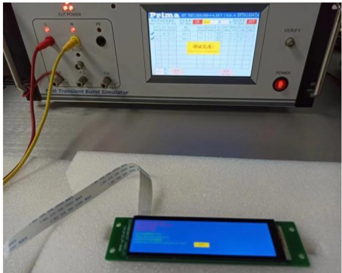
图 3-4 群脉冲测试图
